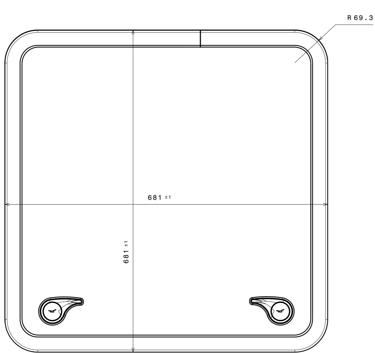
Vue de face Echelle : 1:5
